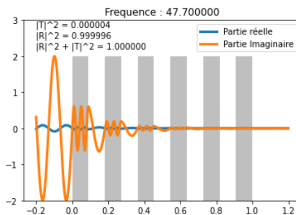
FIGURE 13 – bande interdite pour n=11
