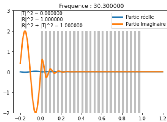
FIGURE 14 – bande interdite pour n=50
